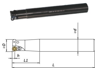
Пластина RPMW/T1204 M0
